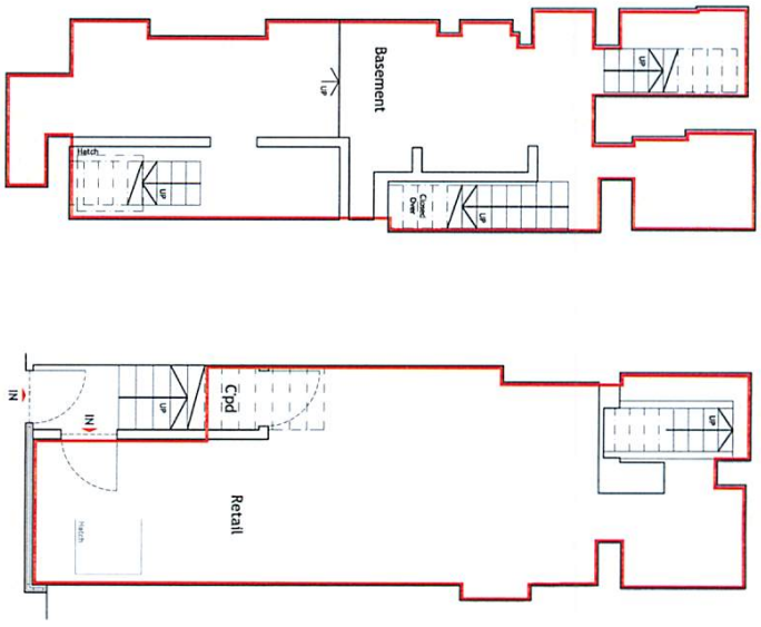
-01 Basement Plan 1:100
